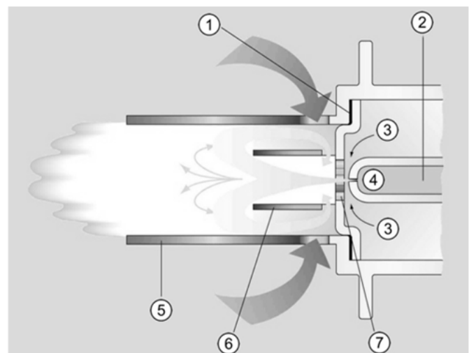
Abb. 52: Verbrennungsablauf Raketenbrenne®
