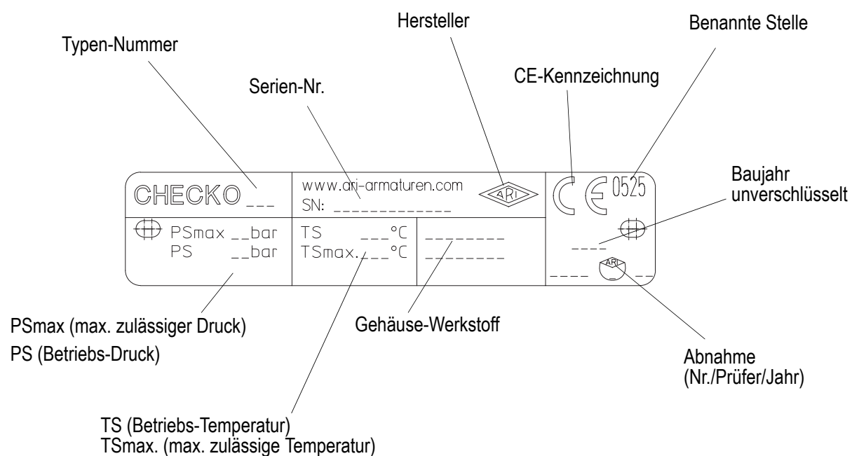
Bild 8: Typenschild
