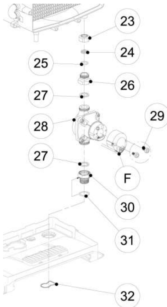
Abb. 88: Umwälzpumpe mit Verschraubungen
