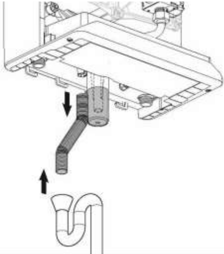
Abb. 78: Demontage des Kondensatschlauchs
