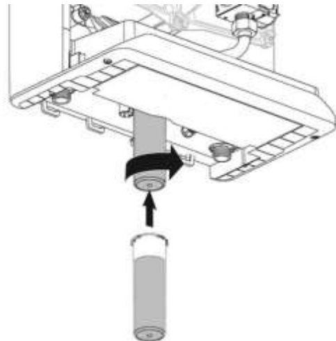
Abb. 85: Montage der Siphontasse
