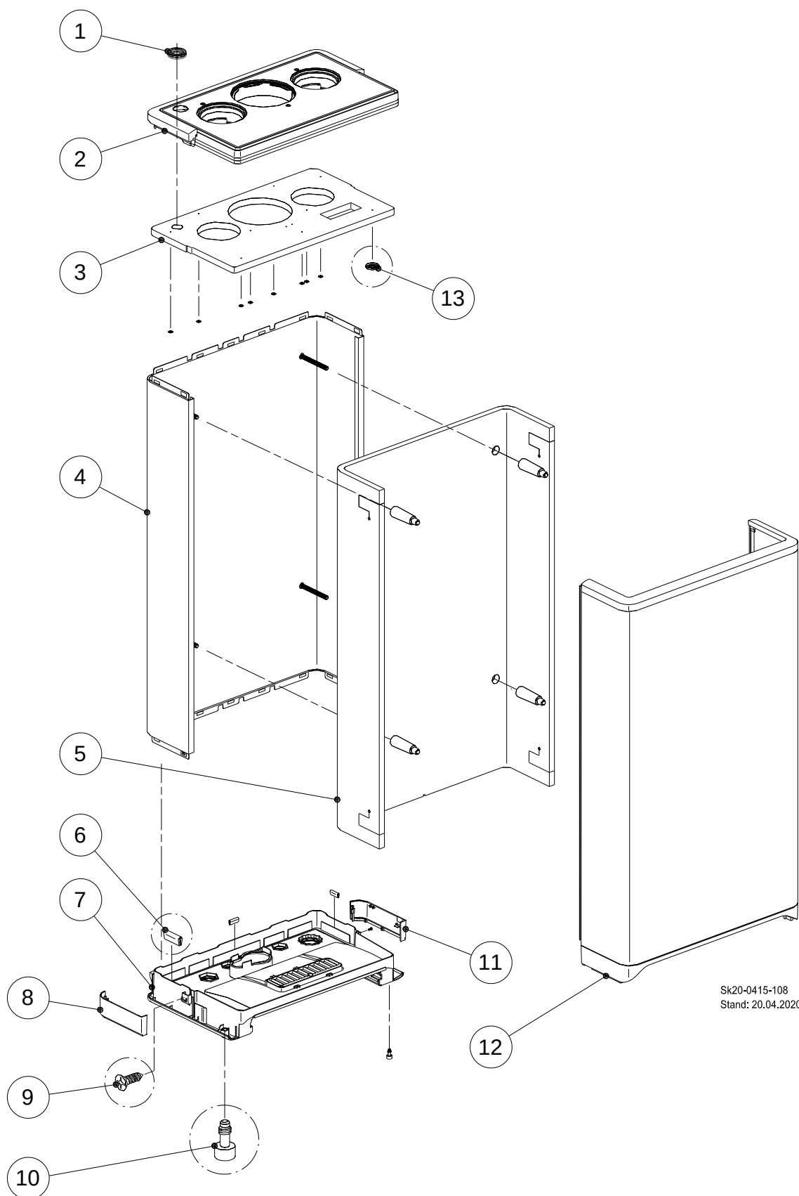
Abb. 91: Verkleidung
