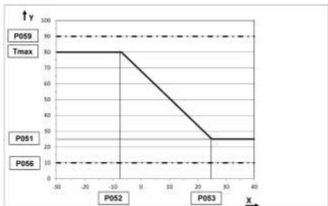
Abb. 69: Heizkennlinie gemäß Werkseinstellungen
