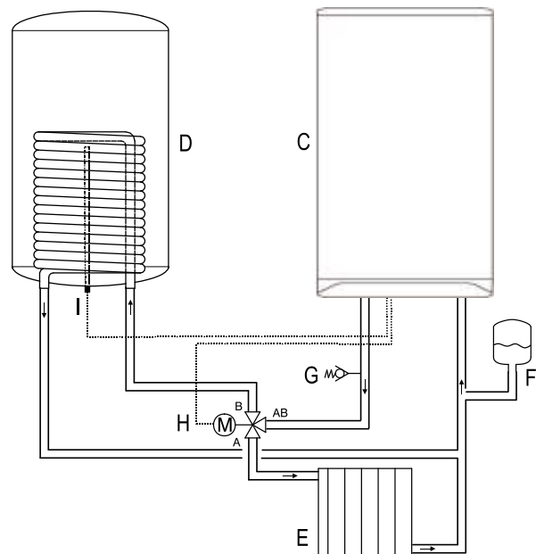
Abb. 22: Trinkwarmwasserbereitung mit externem Speicher über 3-Wege-Umschaltventil
