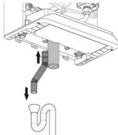
Abb. 86: Montage Kondensatschlauch
