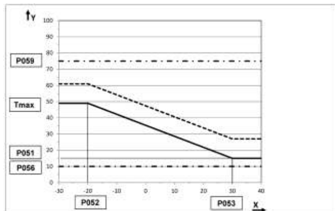
Abb. 71: Heizkennlinie mit Parallelverschiebung ( T_{\text{RaumSoll}} = 24^{\circ}\text{C} , P054 = 3 )
