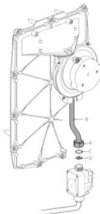
Abb. 73: Umbau Gasdüse
