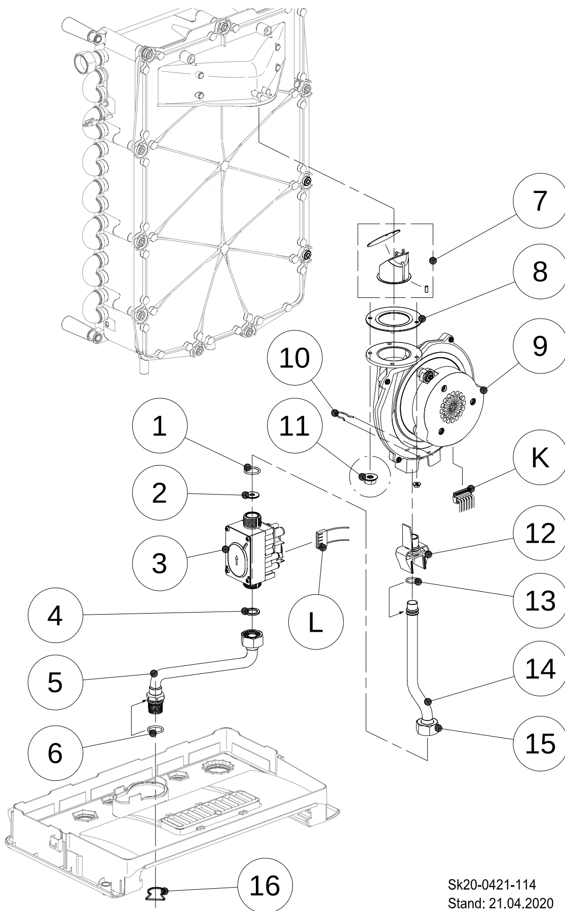
Abb. 95: Gasarmatur und Gebläse
