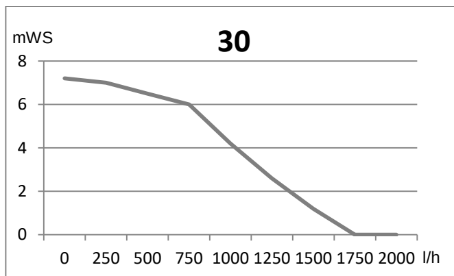
Abb. 103: Restförderhöhe ecoGAS Pro 30, ProX 30/38
