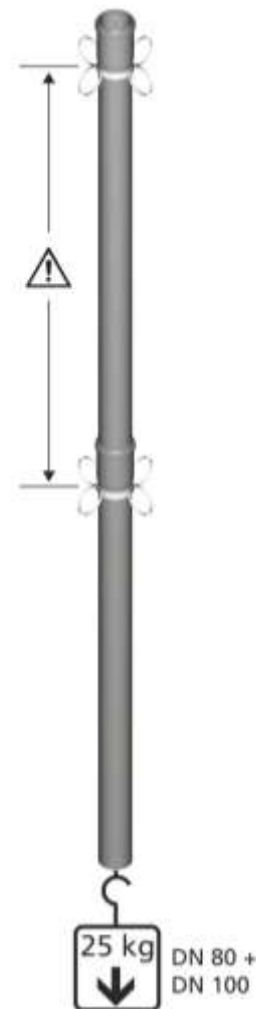
Abb. 41: Abgasrohre mit Stopping-Technik ①
