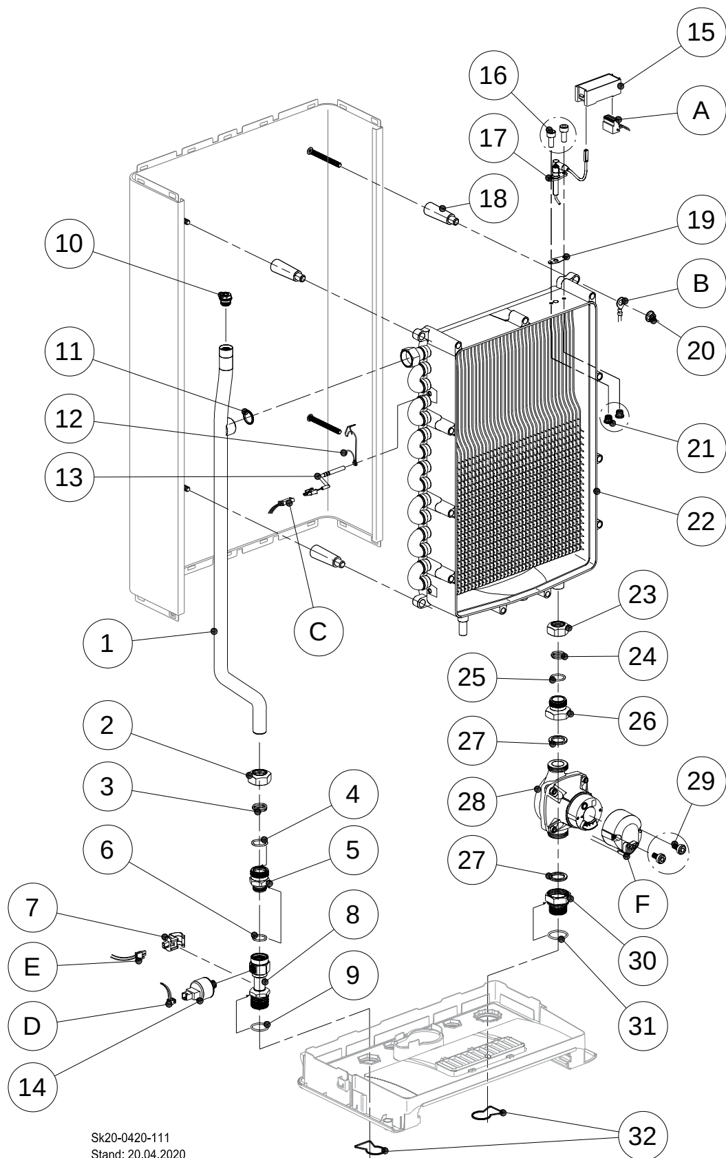
Abb. 92: Wärmetauscher mit Hydraulik Heizkreis
