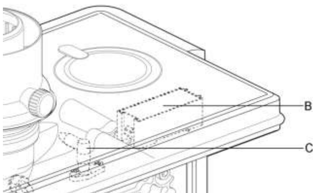
Abb. 87: Zündeinheit B mit Zündelektrode C
