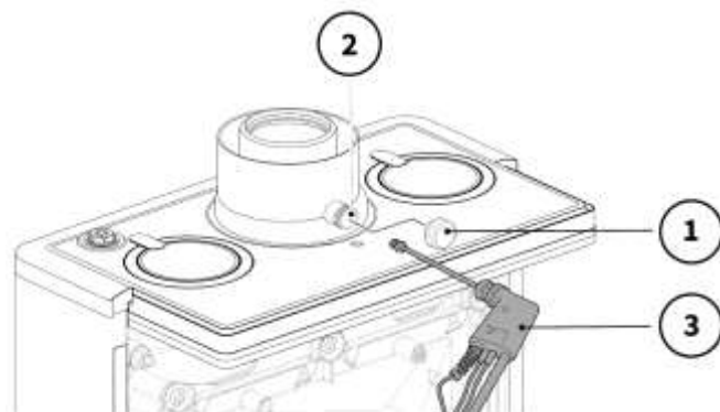
Abb. 75: Mess-Stelle ② am Abgasanschluss
