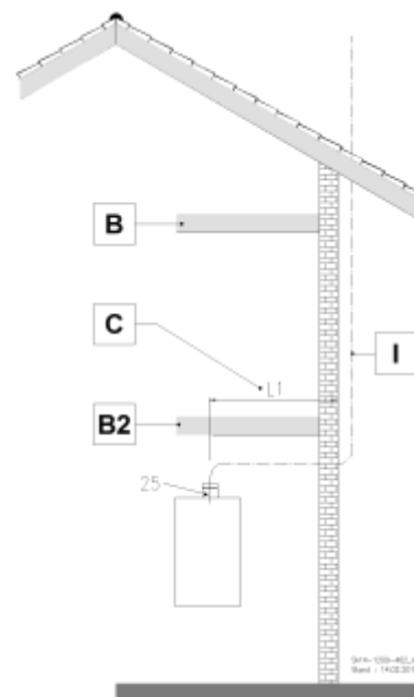
Abb. 35: C 63x Für Anschluss an eine nicht mit der Gasfeuerstätte geprüfte Verbrennungsluftzuführung und Abgasabführung
