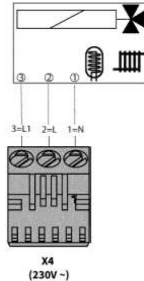
Abb. 21: Anschluss 3-Wege-Umschaltventil
