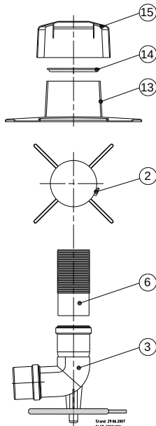
Abb. 47: Detail-Zeichnung Befestigung Schachtabdeckung
