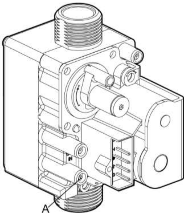
Abb. 56: Gasarmatur
