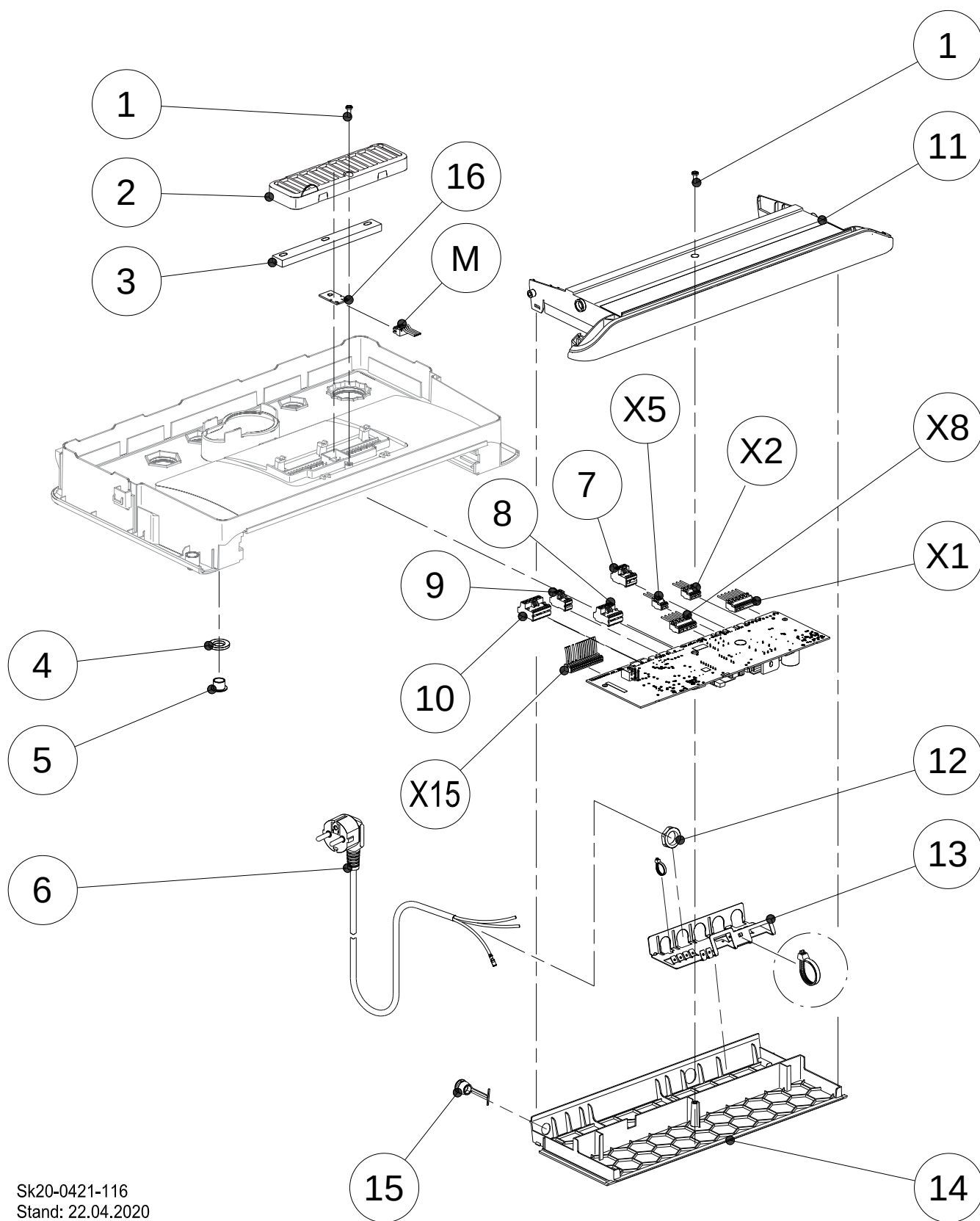
Abb. 97: Regelung und Elektrik
