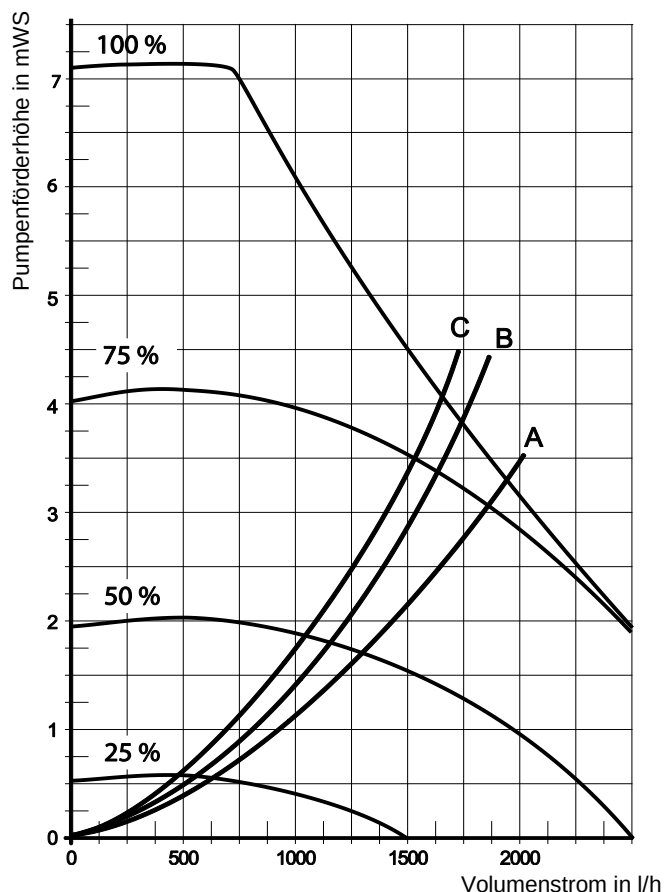
Abb. 68: Hydraulischer Druckverlust des Wärmetauschers auf der Heizungsseite
