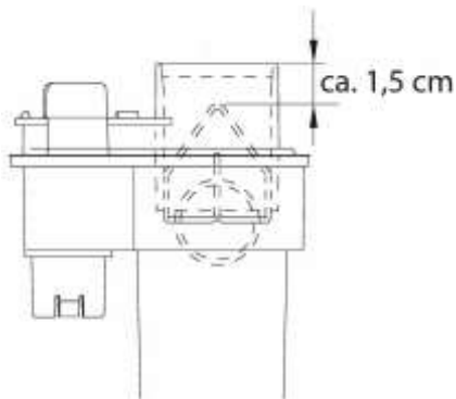
Abb. 82: Korrekte Position von Sicherungsklammer und Kunststoffkugel
