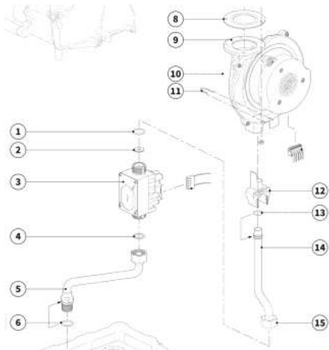
Abb. 76: Komponenten des Gas-Luft-Verbundes
