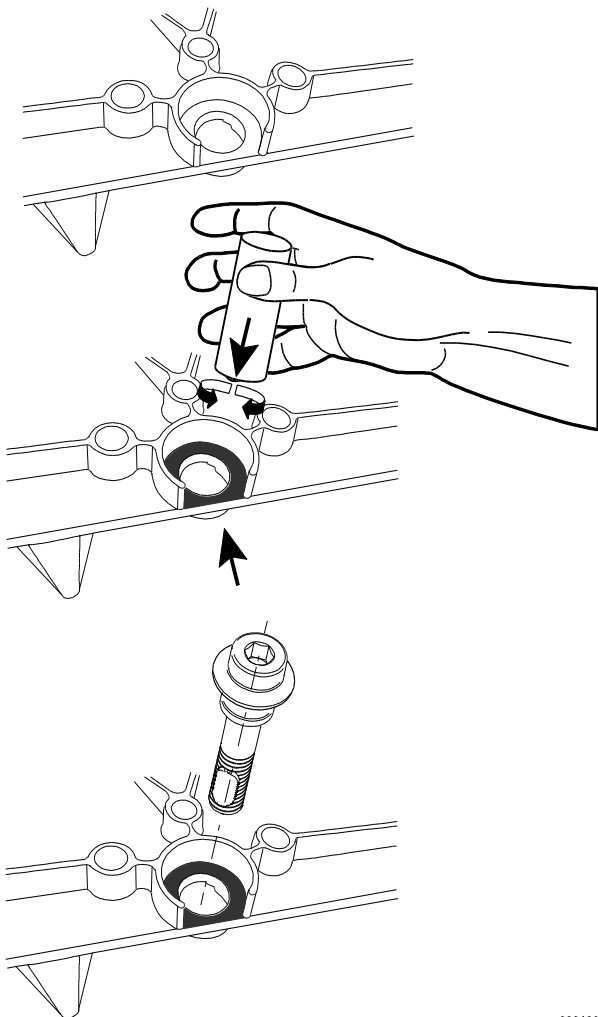
Abb. 89: Auftragen der Keramikpaste (Sach-Nr. 96.38564-7202)
