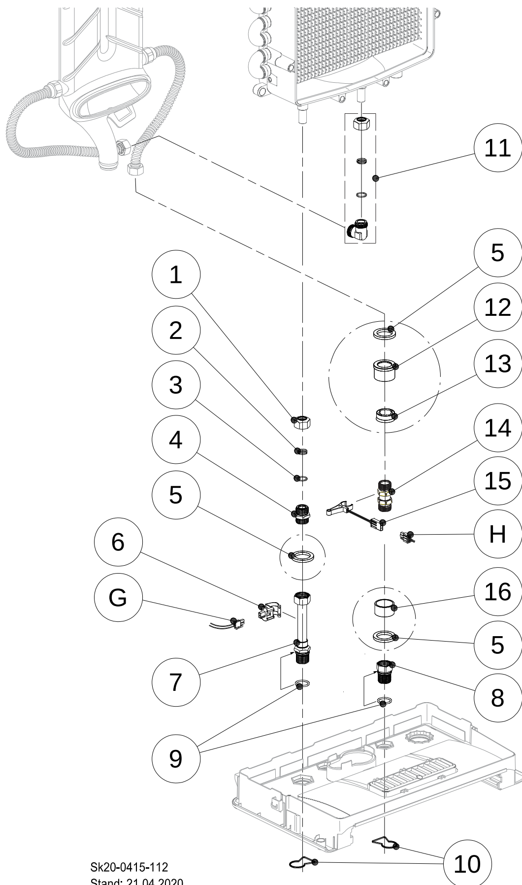
Abb. 93: Hydraulik Trinkwasser
