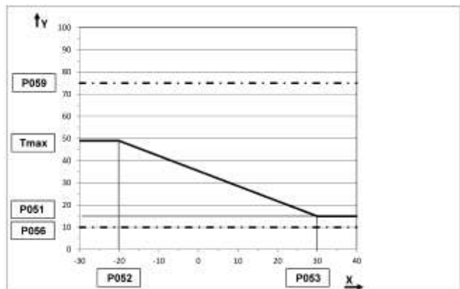
Abb. 70: Heizkennlinie mit geänderten Einstellungen
