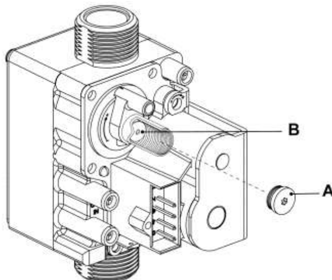
Abb. 77: Gasventil
