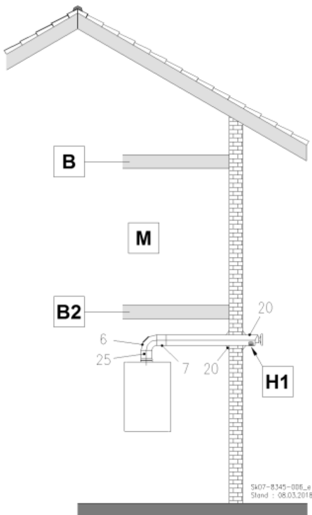
Abb. 30: C 13x Luft-Abgas-Rohrsystem horizontal durch die Außenwand
