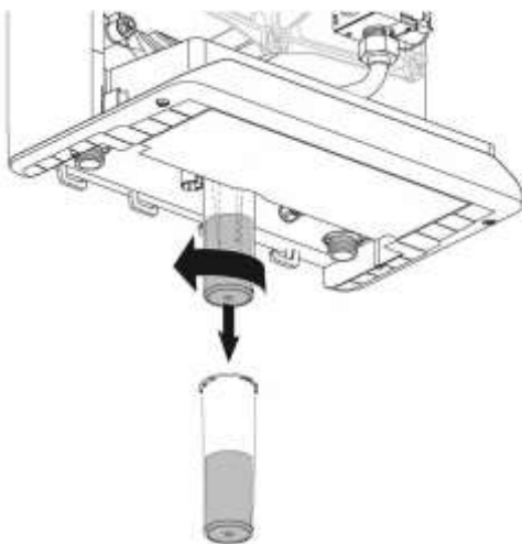
Abb. 79: Demontage der Siphontasse
