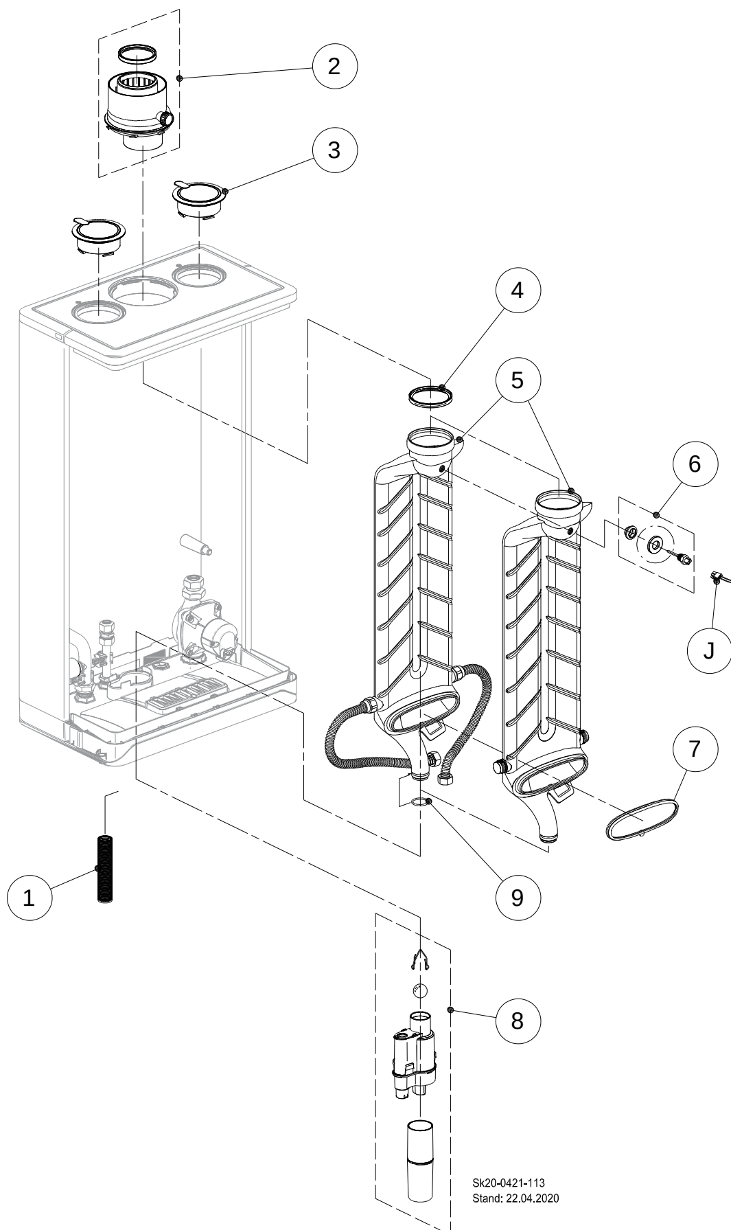
Abb. 94: Abgas und Kondensat
