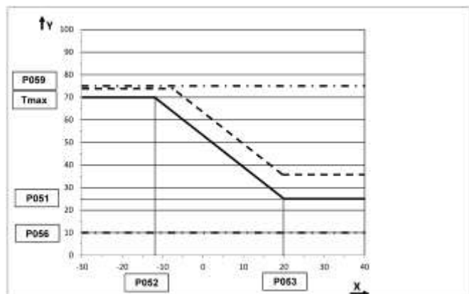
Abb. 72: Heizkennlinie mit Parallelverschiebung ( T_{\text{RaumSoll}} = 24^\circ\text{C} , P054 = 3 ) und Begrenzung durch Parameter P059
