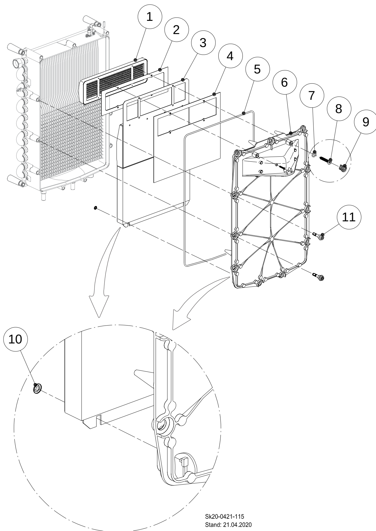
Abb. 96: Brennereinheit
