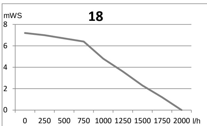
Abb. 101: Restförderhöhe ecoGAS Pro 18, ProX 18/24
