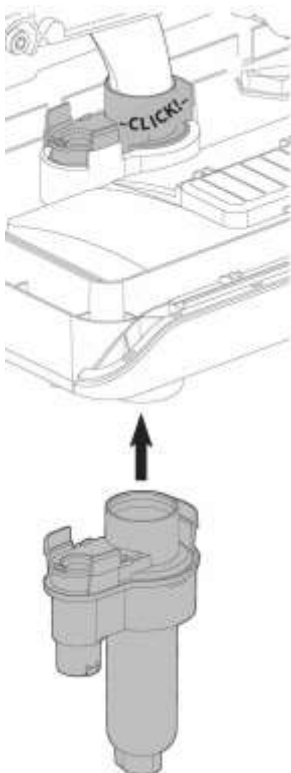
Abb. 83: Montage des Siphons
