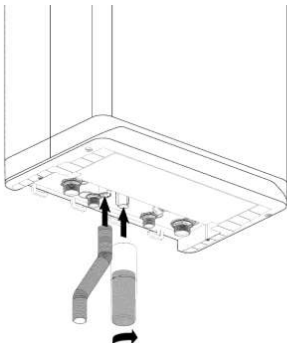
Abb. 8: Montage der Siphontasse und des Kondensatschlauchs
