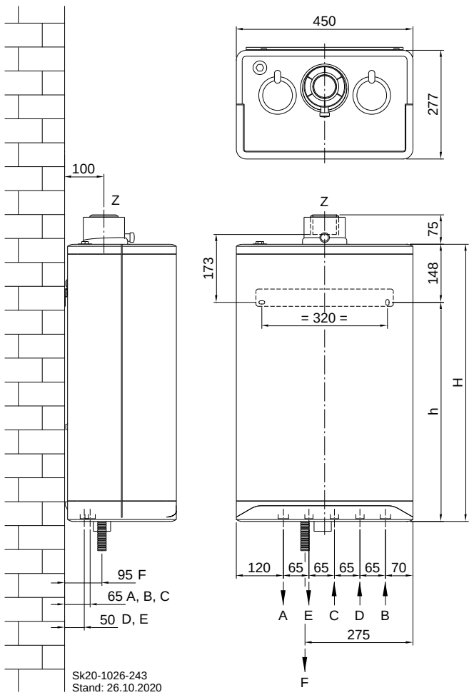
Abb. 4: Gerät mit Wandschiene
