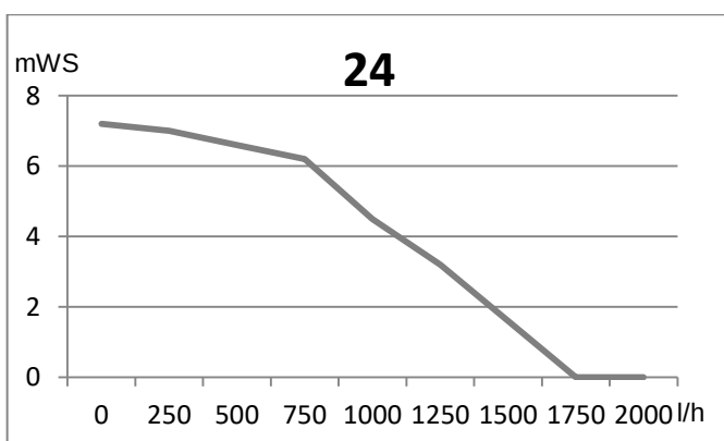
Abb. 102: Restförderhöhe ecoGAS Pro 24
