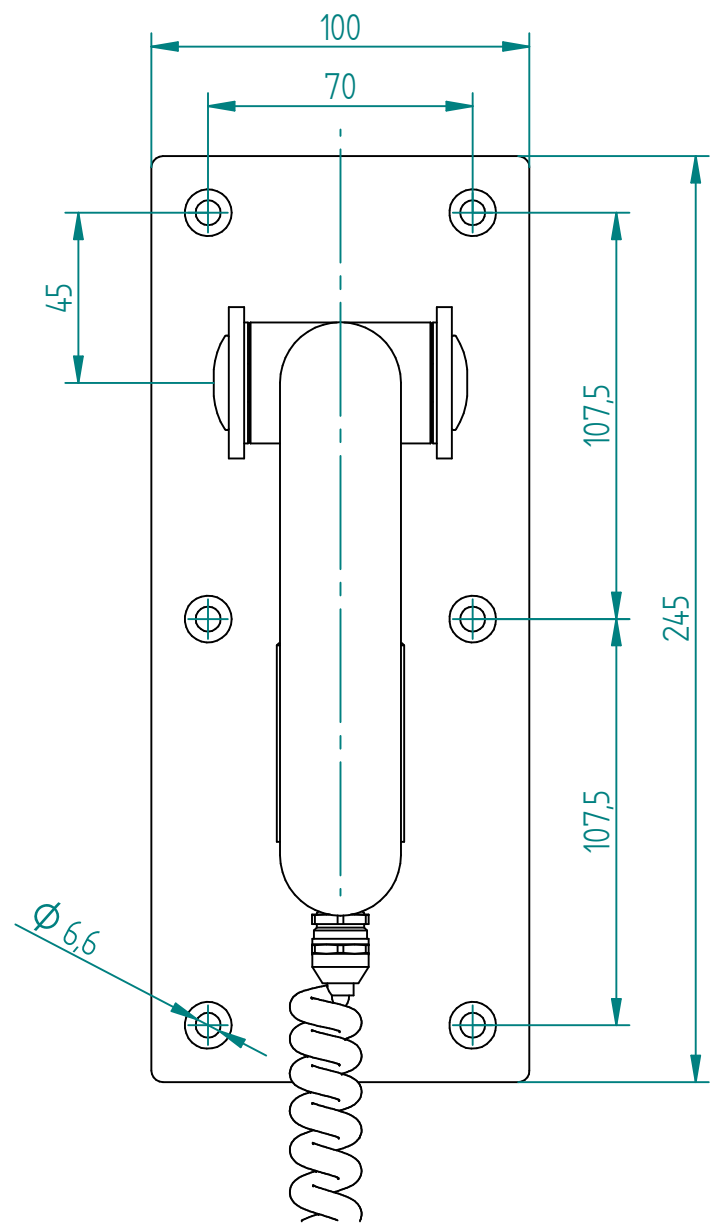
Montageskizze & Bohrbild
