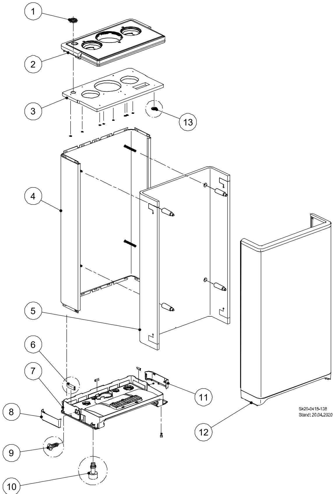
Abb. 109: Verkleidung
