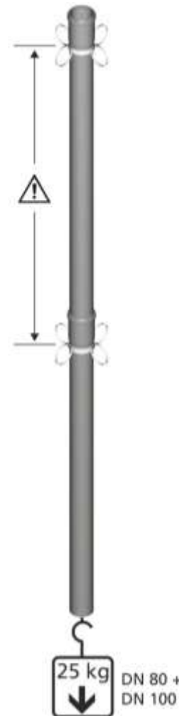
Abb. 41: Abgasrohre mit Stopping-Technik ①
