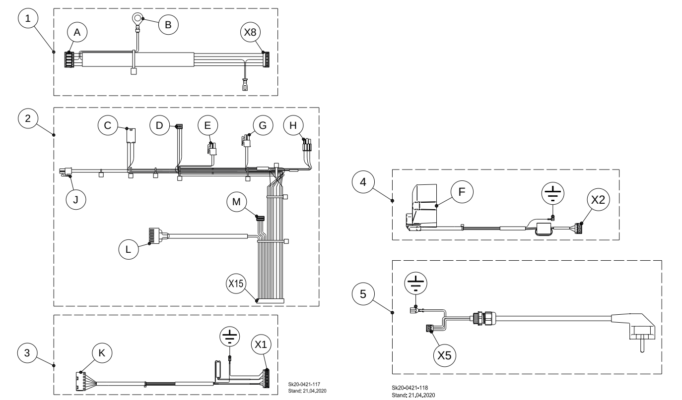
Abb. 98: Verdrahtung
