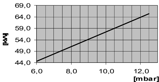
Abb. 25: Leistungsdigramm RE 1.60 H
