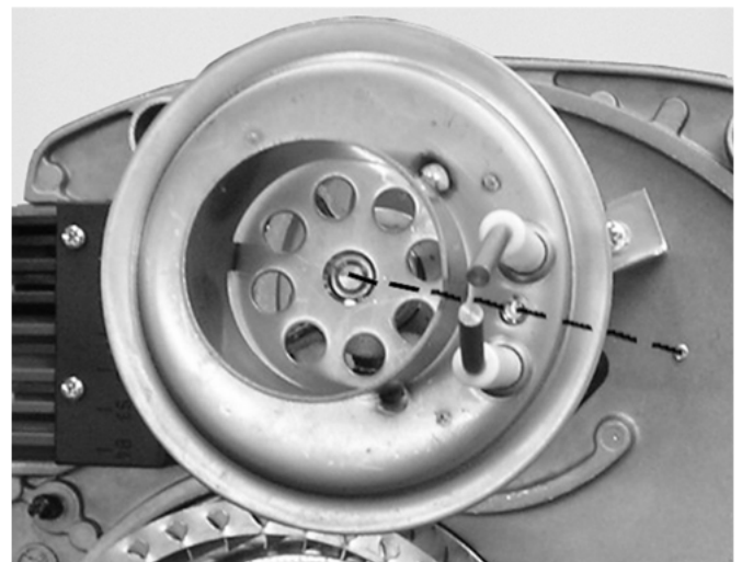
Abb. 40: Mischsystempositionierung und Ausrichtung Zündelektrode
