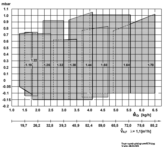
Abb. 50: Arbeitsfeld der Raketenbrenner® RE 1H / HK / HG
