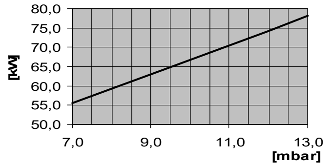
Abb. 26: Leistungsdigramm RE 1.70 H
