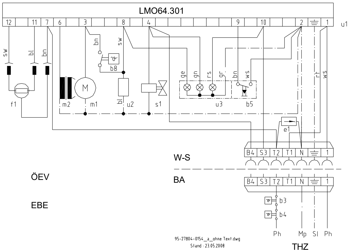
Abb. 14: Schaltplan mit Gebläsenachlauf für RE 1 HG
