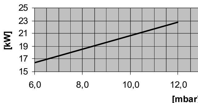
Abb. 19: Leistungsdiagramm RE 1.22 H
