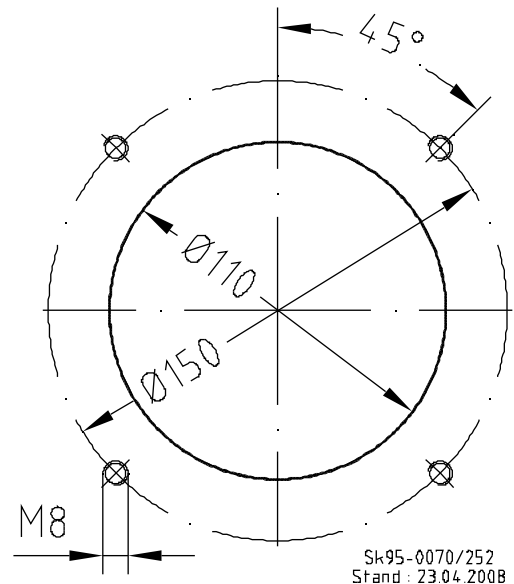
Abb. 5: Kesselanschluss nach DIN EN 226
