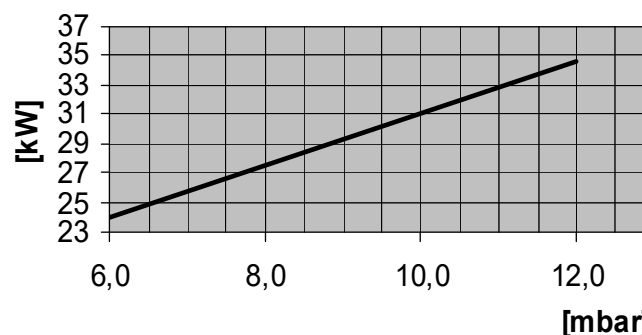
Abb. 21: Leistungsdiagramm RE 1.32 H
