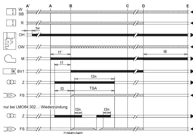
Abb. 33: Programmablauf LMO 64.301 mit Nachlüftungsfunktion (RE 1 HG)
