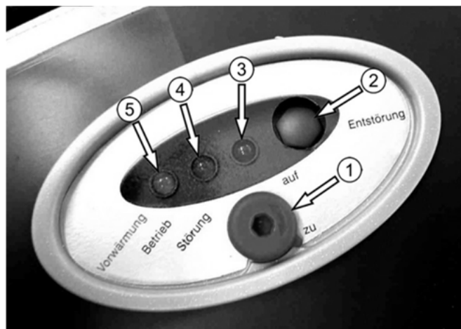
Abb. 15: Lampenfeld RE 1H / RE 1HK / RE 1 HG
