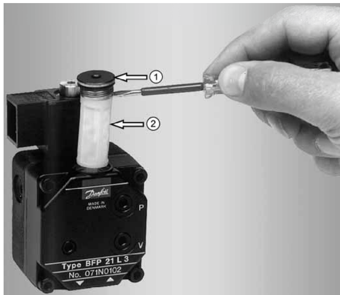
Abb. 46: Herausziehen des Patronenfilters
