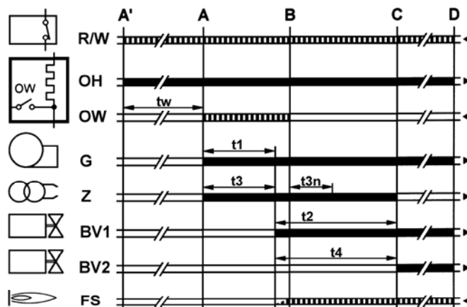
Abb. 32: Programmablauf LMO 44.255 (optional für WLE-Ausführung)
