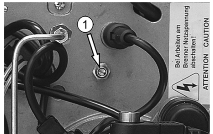
Abb. 27: Messnippel ① zur Prüfung der Gebläsepression
