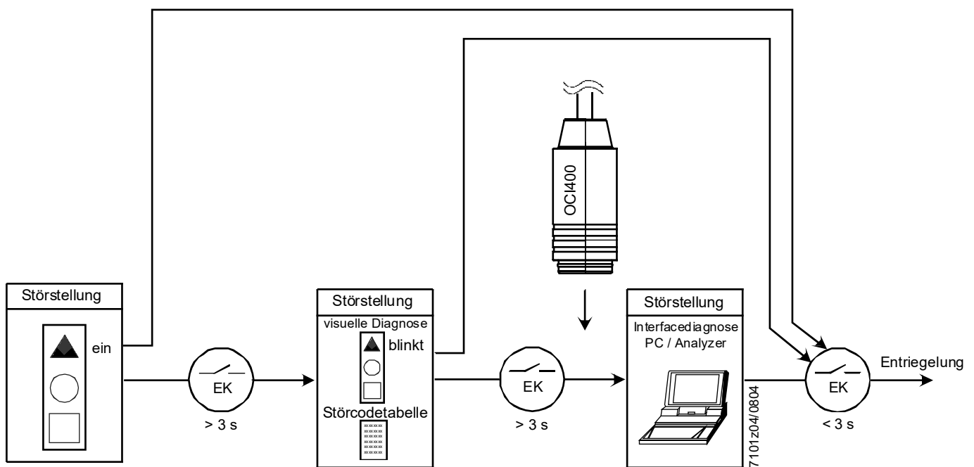
Abb. 48: Ablauf Störursachendiagnose EK = Entriegelungstasters
