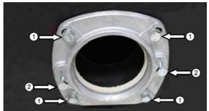
Abb. 6: Befestigung Kesselflansch
