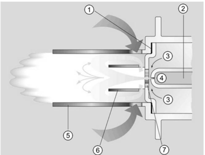
Abb. 52: Verbrennungsablauf Raketenbrenner®
