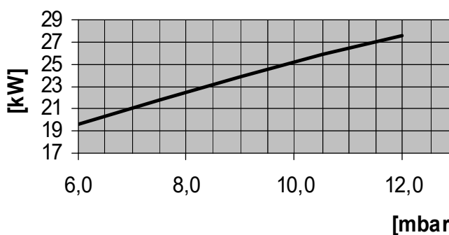
Abb. 20: Leistungsdiagramm RE 1.26 H
