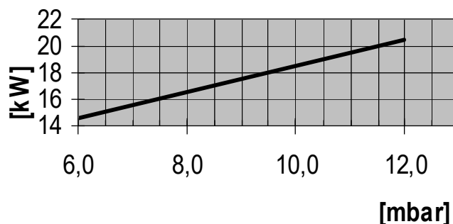
Abb. 18: Leistungsdiagramm RE 1.19 H
