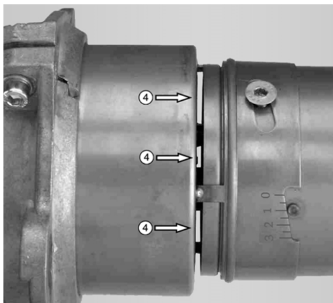
Abb. 9: Rezirkulationsschlitze ④
