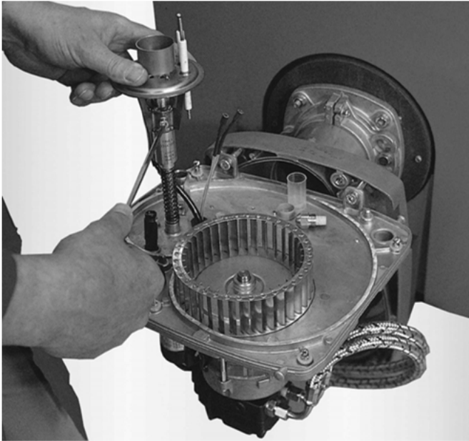
Abb. 37: Demontage Mischsystem
