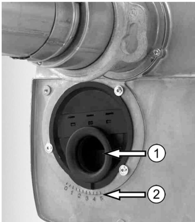
Abb. 30: Lufteinlaufdüse ① und Skala ②
