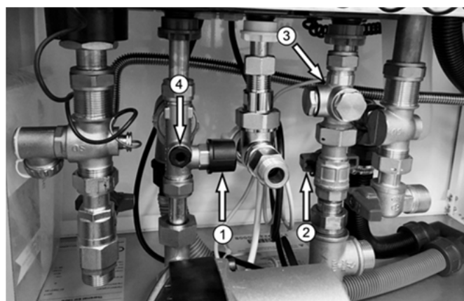
Abb. 90: Spülanschlüsse der Trinkwarmwasserschlange beim Kompakt
