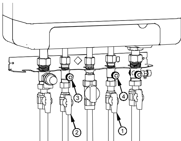
Abb. 89: Spülanschlüsse der Trinkwarmwasserschlange beim Kombi
