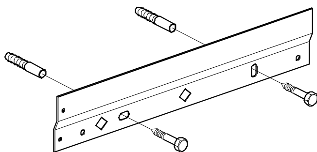
Abb. 8: Wandschiene
