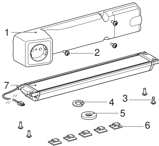
Kuva 1: Geberit-pistorasia, jossa on ComfortLight-moduuli
