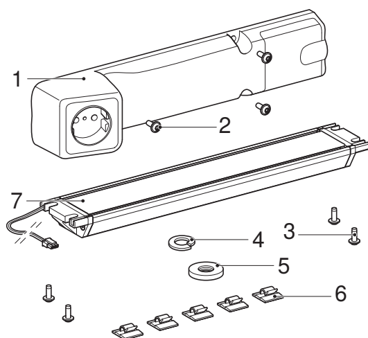
Slika 1: Element z vtičnico Geberit z modulom ComfortLight
