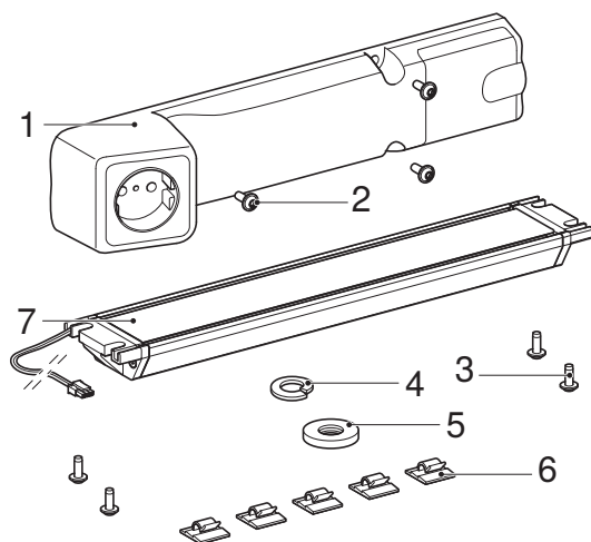
Зображення 1: Розетковий блок Geberit із модулем ComfortLight
