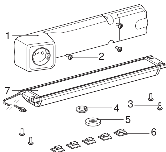
Abbildung 1: Geberit Steckdosenelement mit ComfortLight-Modul
