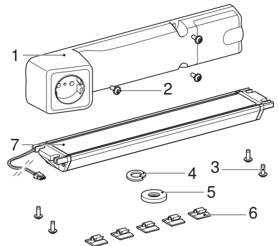
الشكل 1: عنصر مقبس Geberit مع وحدة ComfortLight
