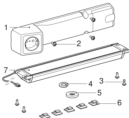
Joonis 1: Geberiti pistikupesa element koos ComfortLighti mooduliga
