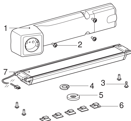
1. Attēls: Geberit kontaktligzdas elements ar ComfortLight moduli
