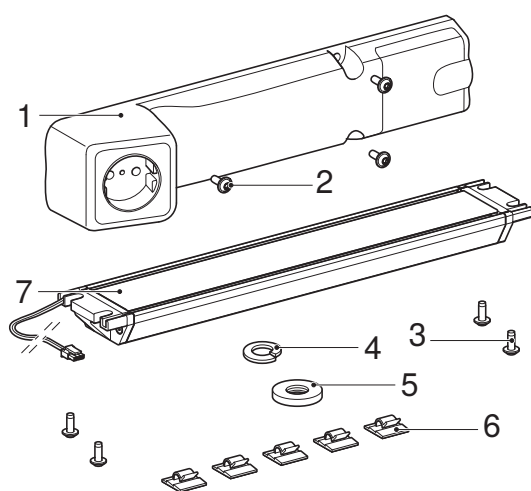
插图 1: 带 ComfortLight 模块的 Geberit 插座元件
