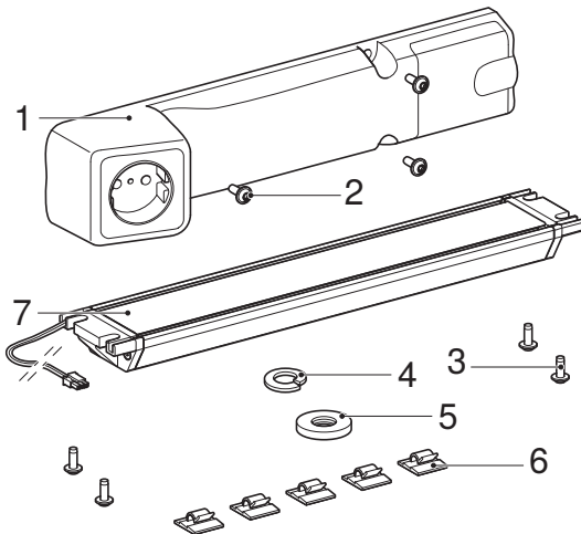
Şekil 1: ComfortLight modüllü Geberit priz ünitesi
