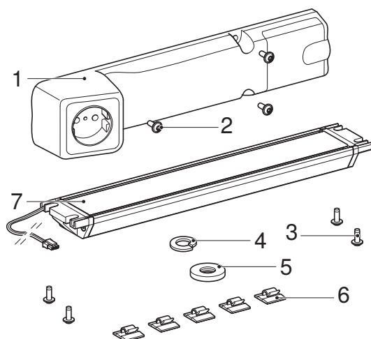
Εικόνα 1: Προέκταση πρίζας Geberit με μονάδα ComfortLight
