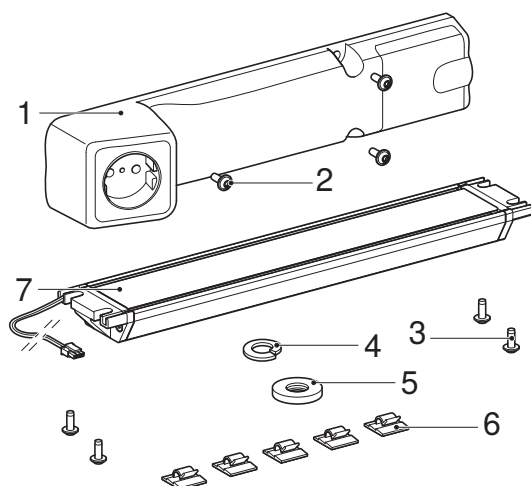
Slika 1: Geberit utičnica sa ComfortLight modulom
