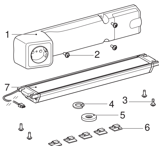
Figura 1: Element de priză Geberit cu modul ComfortLight
