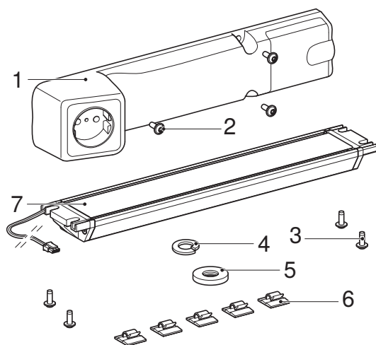
Mynd 1: Geberit tengill með ComfortLight-einingu
