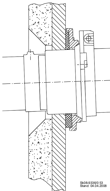
Abb. 10: Konusförmig ausgeschnittene Auskleidung
