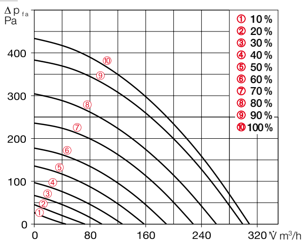
Kennlinie KWL 300 W
