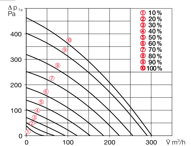
Kennlinie KWL 300 W
