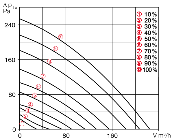
Kennlinie KWL 200 W ET
