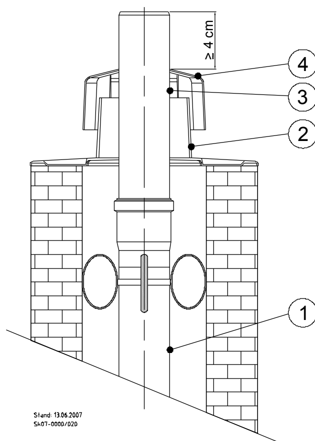
Abb. 42: Schachtabdeckung
