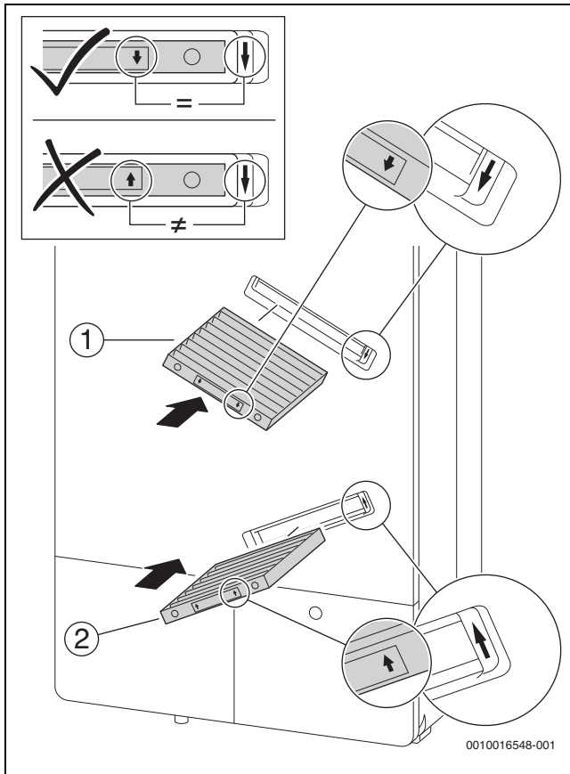
Bild 6 Filter einschieben
