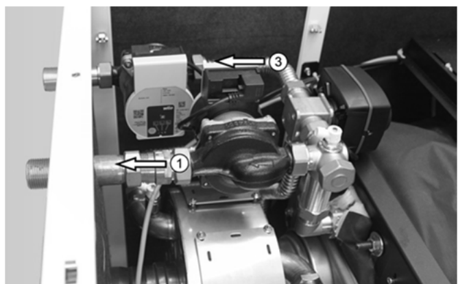
Abb. 14: Vorlauf Direktkreis ① sowie Vorlauf Mischer- kreis ③ (bei Ausführung ecoDUO ..i)
