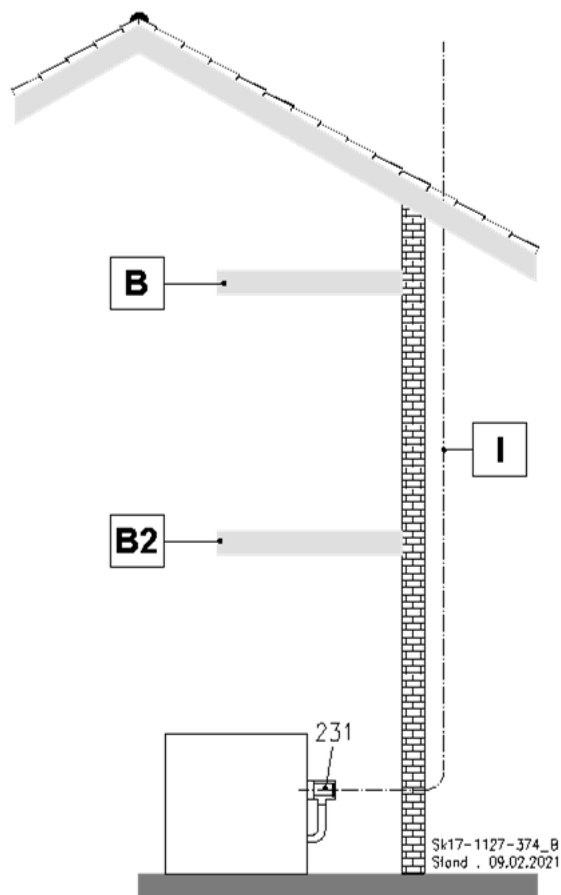
Abb. 34: C 63x Für Anschluss an eine nicht mit der Gasfeuerstätte geprüfte Verbrennungsluftzuführung und Abgasabführung
