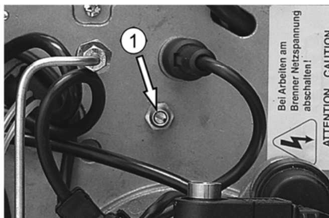
Abb. 16: Messnippel ① zur Prüfung der Gebläsepression
