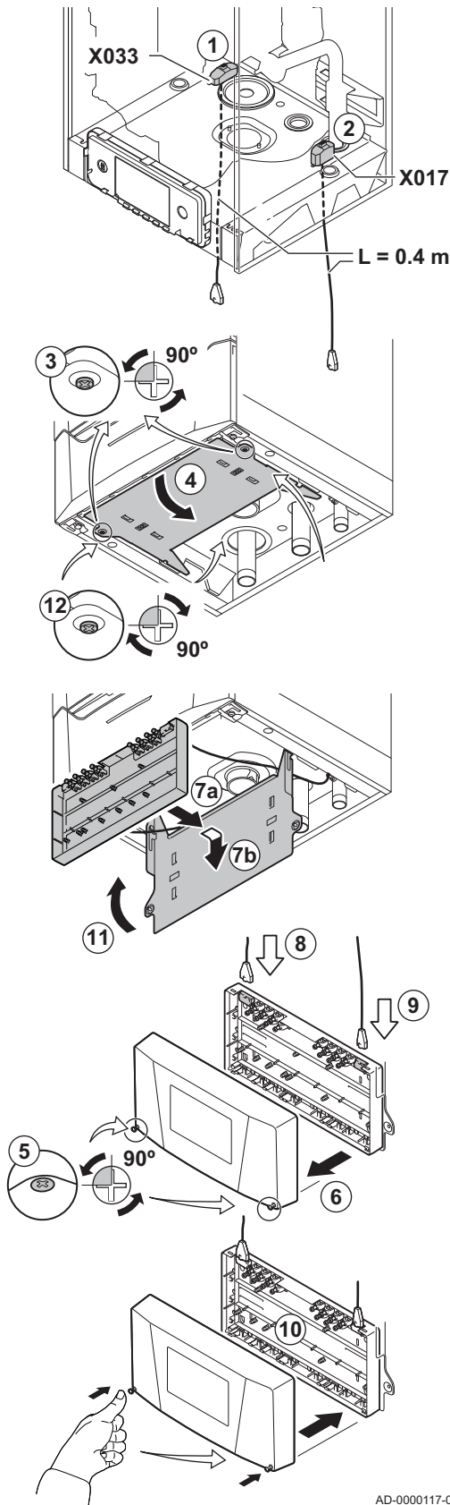
Abb.42 Öffnen der Anschlussdose
