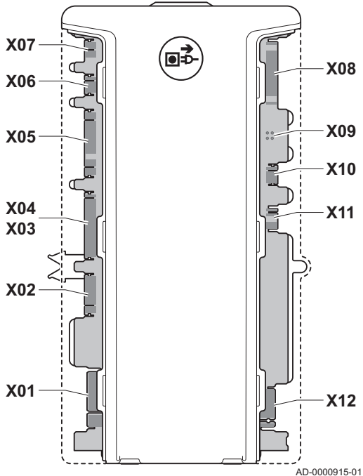
Abb.39 Steckverbinder von der Regelungseinheit CU-GH06 (Frontansicht)
