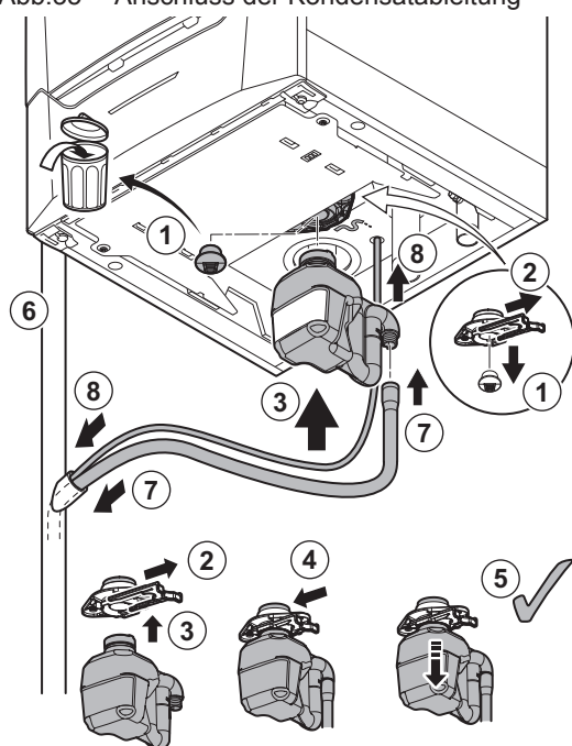
Abb.35 Anschluss der Kondensatableitung
