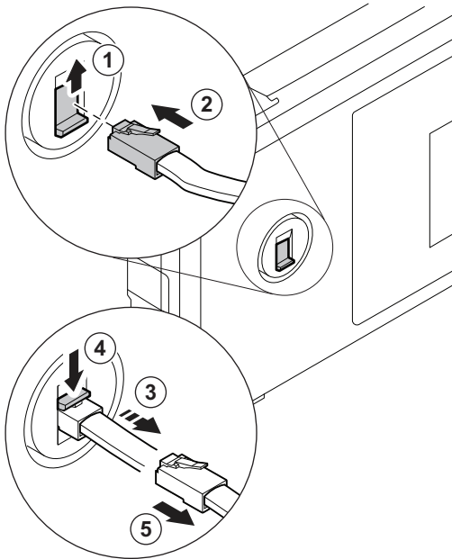
Abb.68 Anschluss eines Schnittstellensteckers
