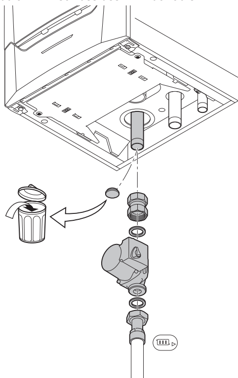
Abb.34 Anschluss des ZH-Rücklaufs
