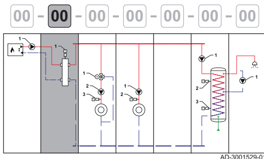
Abb.28 Anschluss
