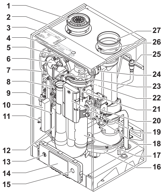
Abb.1 Hauptkomponenten
