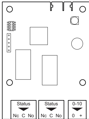
Abb.54 Regelungsleiterplatte SCB-01
