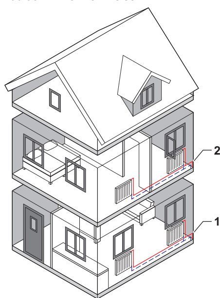
Abb.93 Zwei Heizkreise
