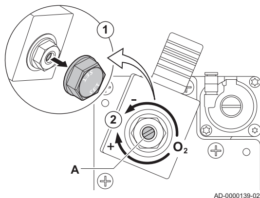
Abb.77 Position der Einstellschraube A
