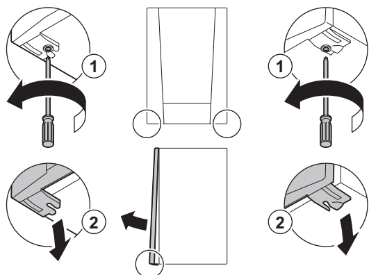
Abb.87 Öffnen des Kessels
