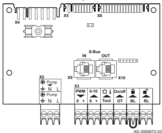
Abb.43 Anschlussleiterplatte CB-01
