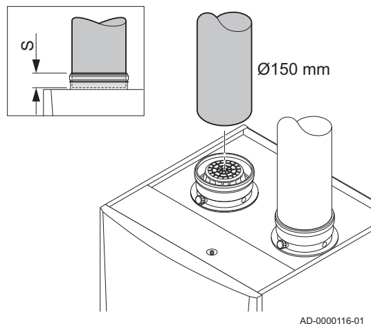
Abb.38 Anschluss der Luftzufuhr
