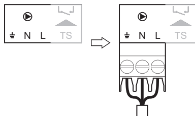
Abb.23 Kombiniertes Steckverbinder
