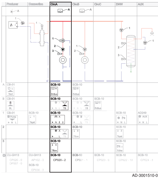
Abb.16 Heizanforderung
