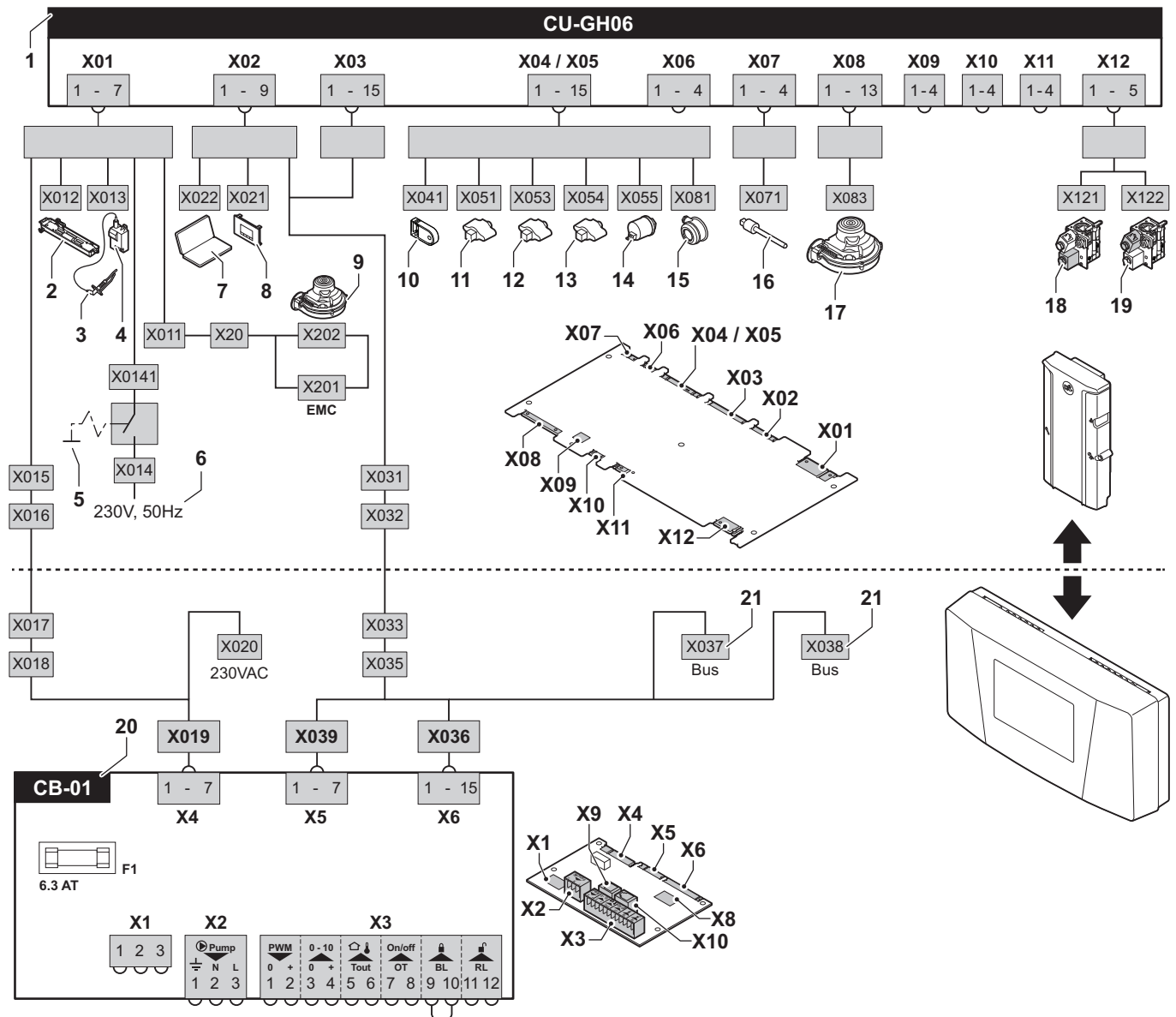
Abb.101 Elektrischer Schaltplan
