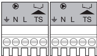
Abb.60 Pumpe mit Schutzthermostatanschluss
