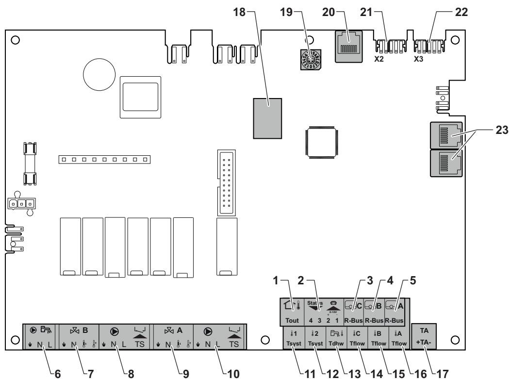
Abb.57 SCB-10 Regelungsleiterplatte
