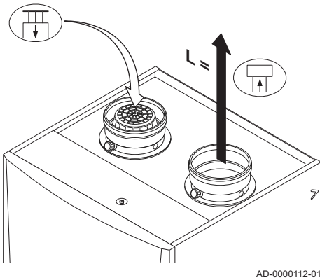
Abb.10 Raumluftabhängige Ausführung
