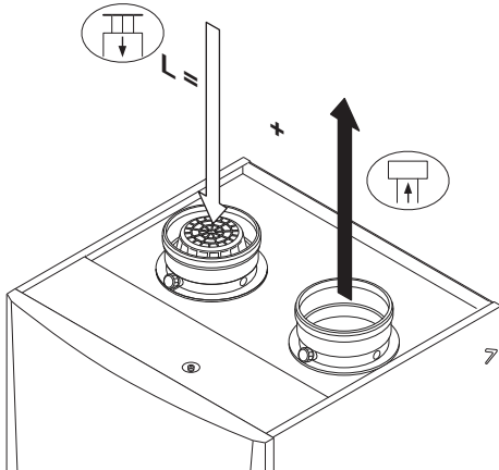
Abb.11 Raumlufunabhängige Ausführung
