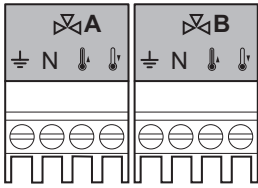
Abb.59 Mischventil-Stecker
