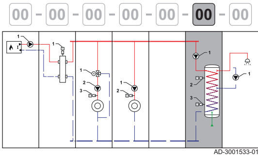
Abb.31 TWW-Erweiterungskreis
