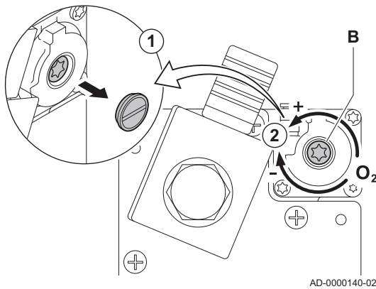
Abb.79 Position der Einstellschraube B
