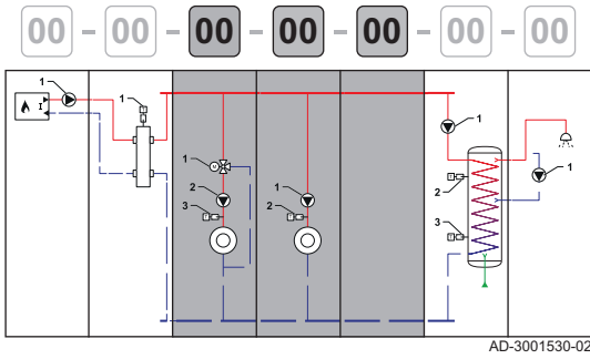
Abb.29 Kreise
