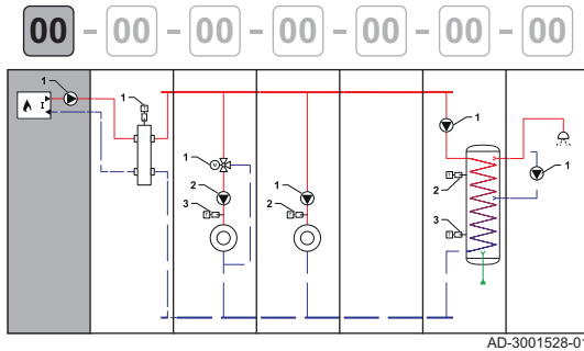
Abb.27 Erzeuger
