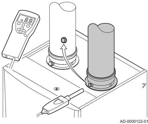
Abb.75 Abgasmesspunkt
