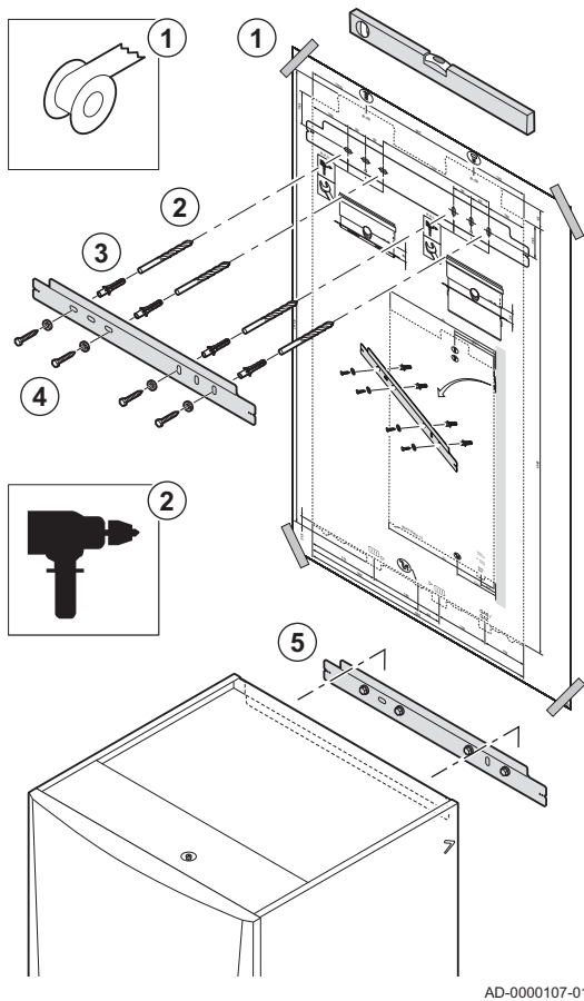
Abb.32 Montage des Heizkessels
