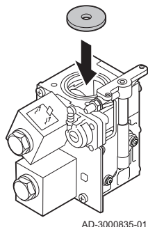
Abb.74 Gasblende einbauen
