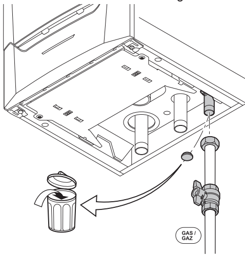
Abb.36 Anschluss der Gasleitung
