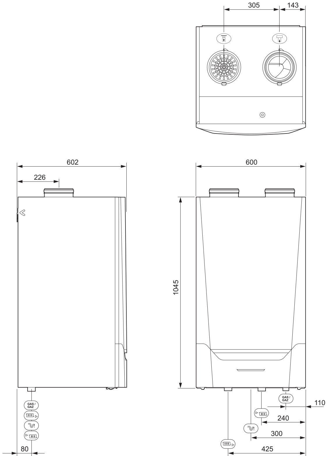
Abb.102 Abmessungen
