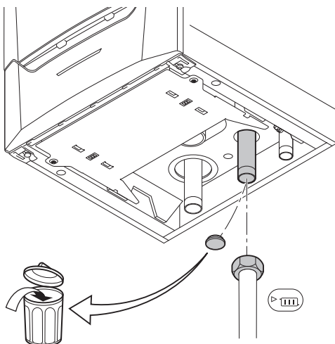
Abb.33 Anschluss des ZH-Vorlaufs
