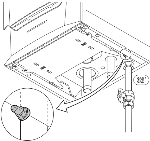
Abb.70 Prüfföffnung für Gas
