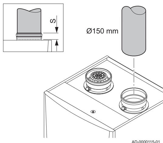
Abb.37 Anschließen des Abgasstutzens
