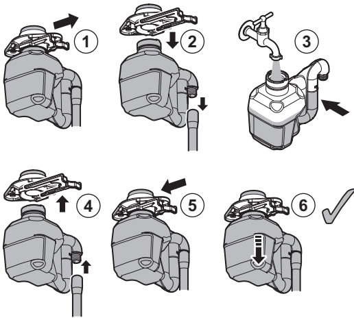
Abb.69 Befüllen des Siphons
