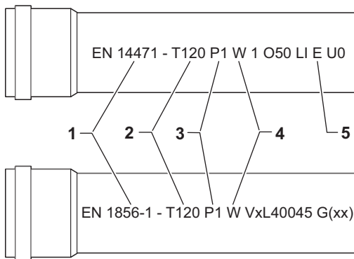
Abb.8 Probestück
