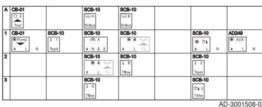
Abb.19 Zu brückende elektrische Anschlüsse
