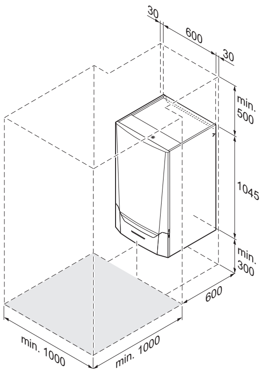
Abb.3 Installationsbereich
